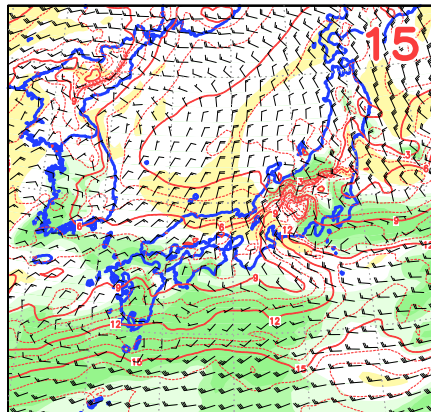
<60>0106UTC T850,TTd850,W850
