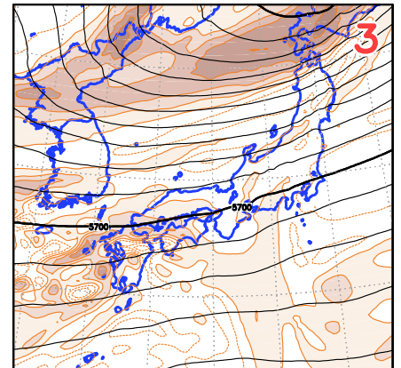
<48>3018UTC Z500 Vor500
