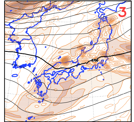
<24>2918UTC Z500 Vor500
