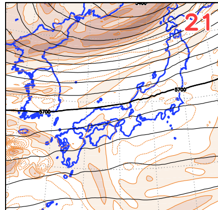
<42>3012UTC Z500 Vor500
