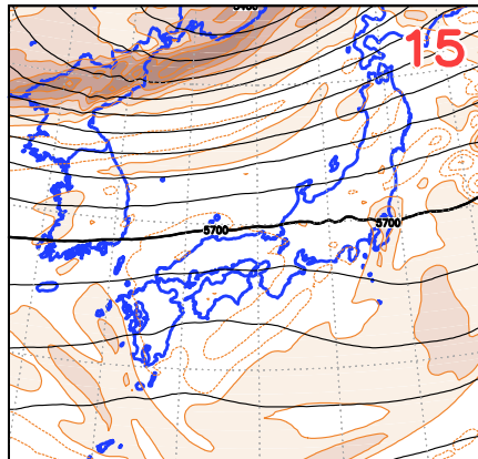
<36>3006UTC Z500 Vor500
