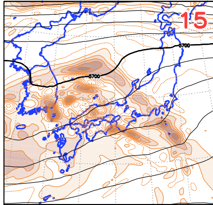
<12>2906UTC Z500 Vor500
