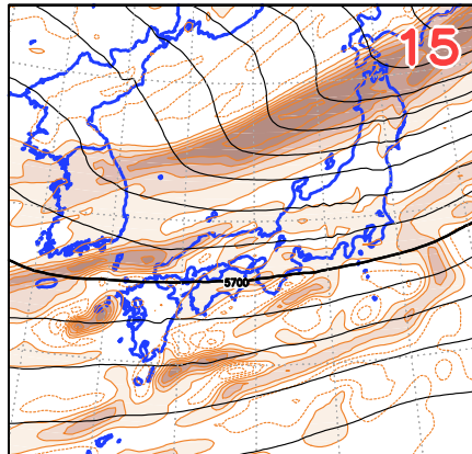
<60>0106UTC Z500 Vor500
