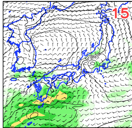
<60>0106UTC Psea Wind R6
