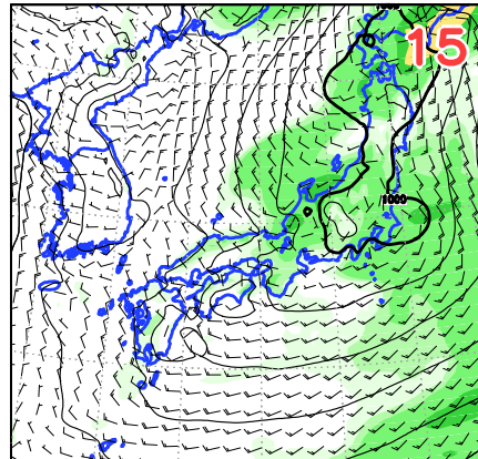
<36>3006UTC Psea Wind R6
